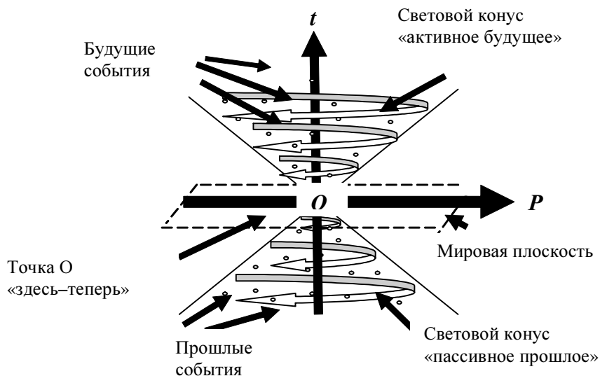
Пространственно-временная диаграмма Минковского.
